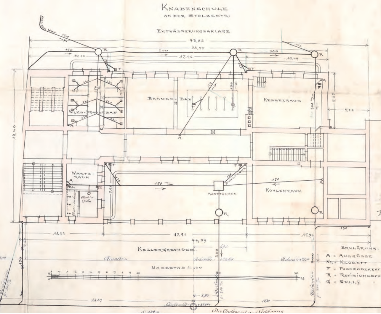
Rycina 62. Rzut piwnic szkoły podstawowej dla chłopców z podłączeniem obiektu do kanalizacji od strony ul. Franciszka Tarczyńskiego, 1908 APS, AMSPB, II/2834
