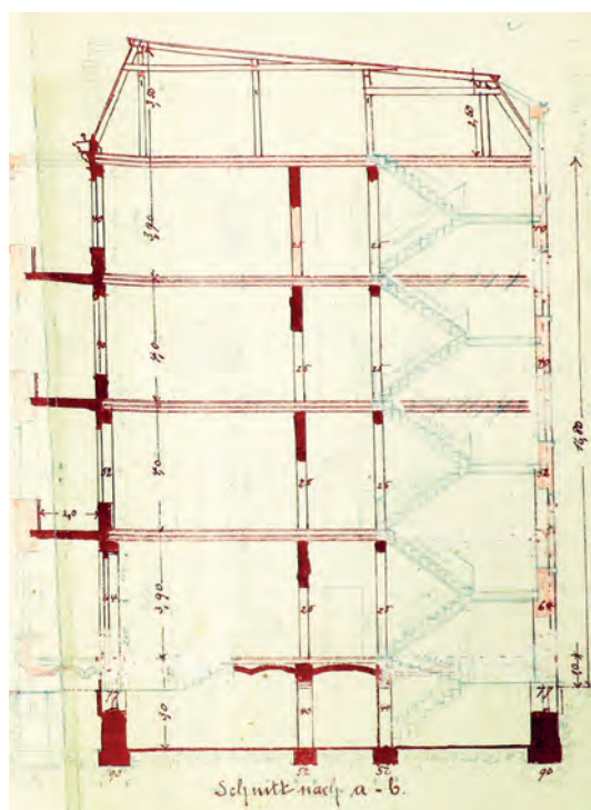
Rycina 16. Przekrój kamienicy, 1892, APS, AMSPB, 48
