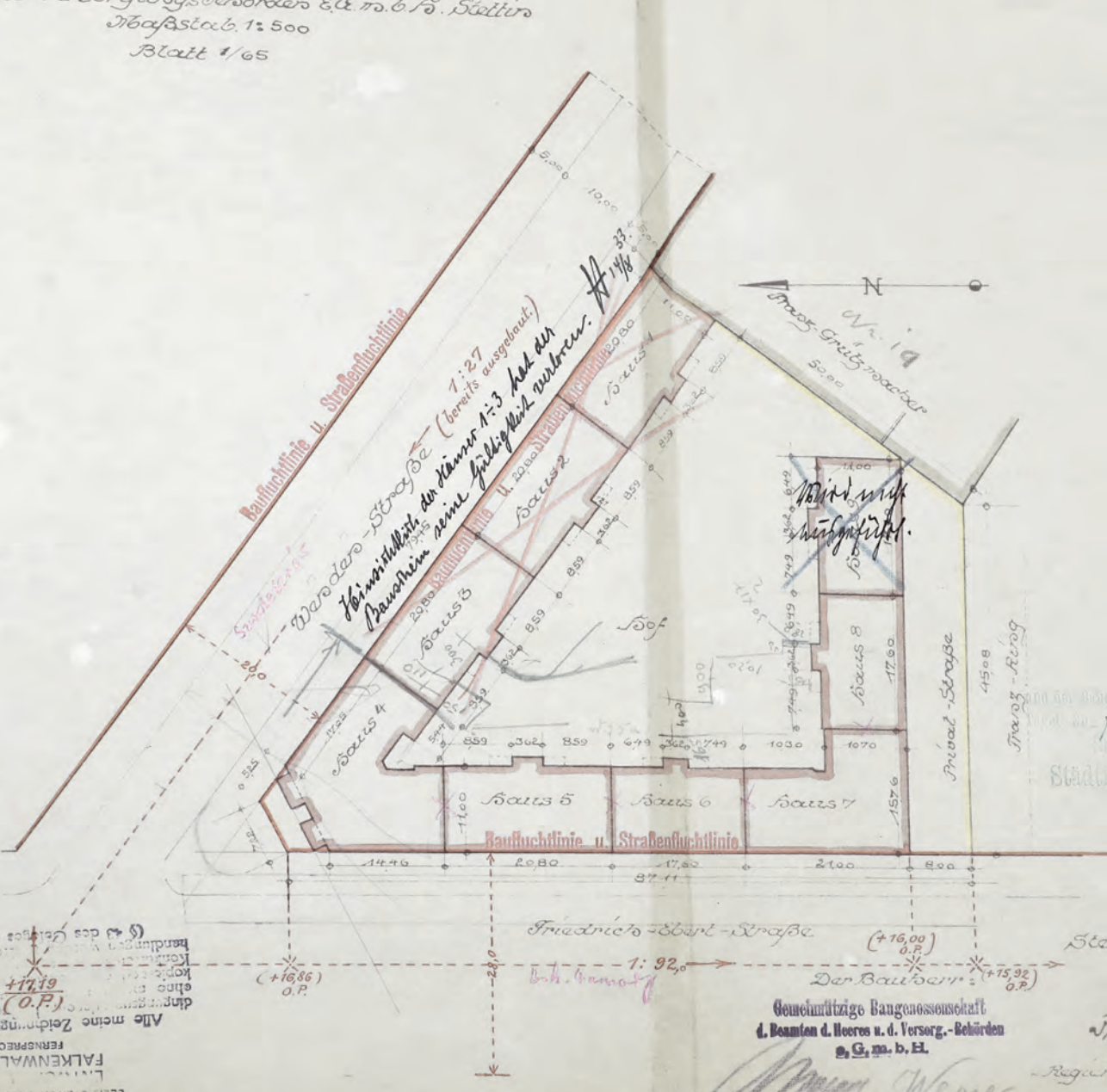
Rycina 66. Budynki mieszkalne i ich położenie na parceli na rogu ul. Szwoleżerów i al. Bohaterów Warszawy (obiekty skreślone nie były realizowane), 1928, APS, AMSPB, 9669
