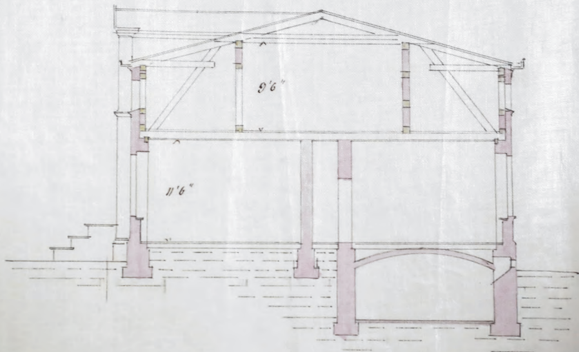
Rycina 78. Przekrój willi Johanna Quistorpa, 1865, APS, AMSPB, 15876
