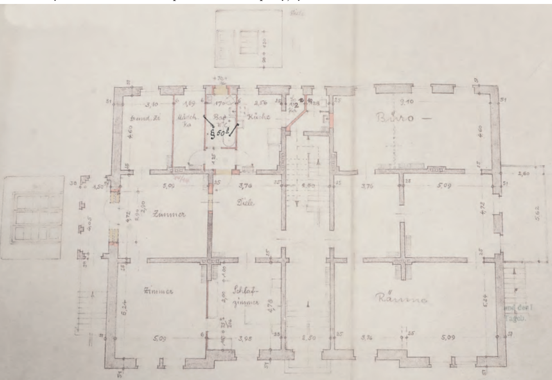
Rycina 59. Parter willi z przeróbkami adaptacyjnymi na cele biurowe, 1932, APS, AMSPB, 6395
