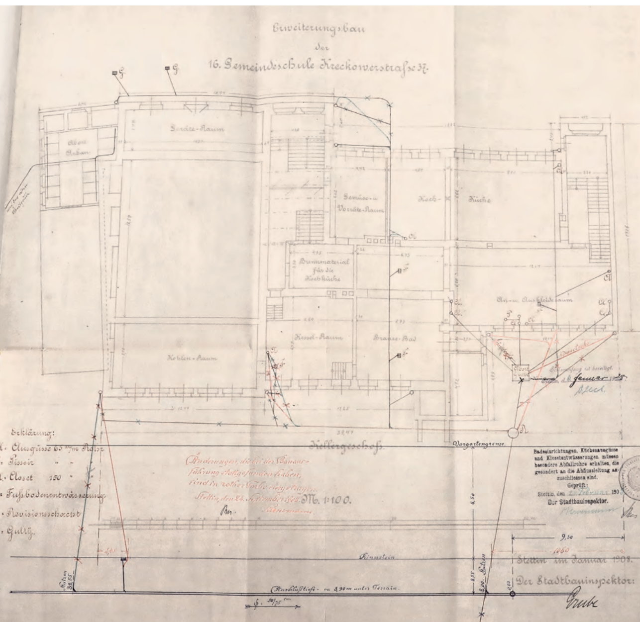
Rycina 48. Rzut piwnic nowej części szkoły podstawowej dla dziewcząt z podłączeniem do kanalizacji od strony ul. Adama Mickiewicza, APS, AMSPB, II/4446
