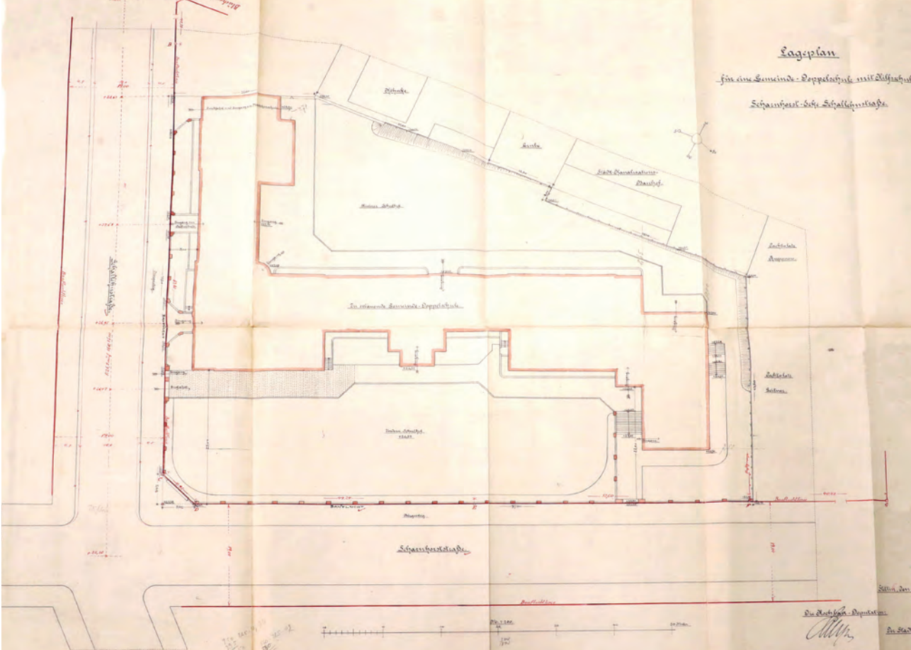
Rycina 44. Położenie budynku Szkoły Podstawowej im. Scharnhorsta na parceli budowlanej róg ulic Unisławy i Wacława Felczaka, 1912, APS, AMSPB, 7159
