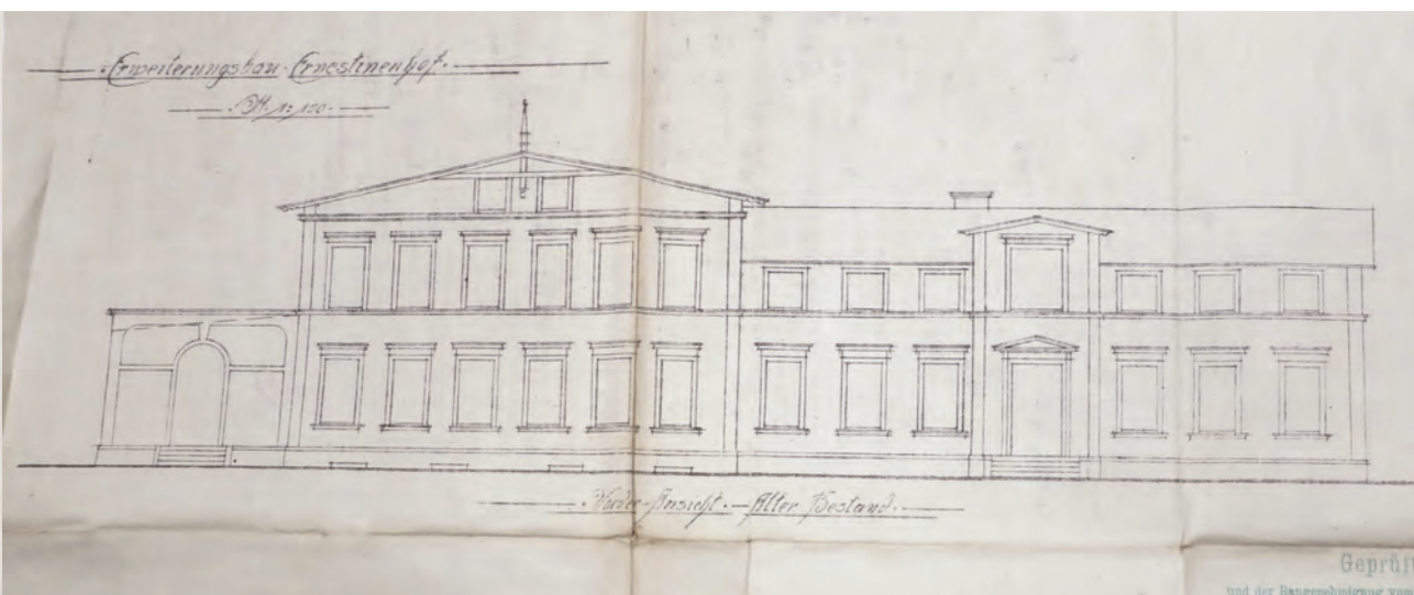
Rycina 85. Elewacja rozbudowanej willi Ernestinenhof z wyraźnie widocznymi częściami starą i nową, 1903 APS, AMSPB, 7900
