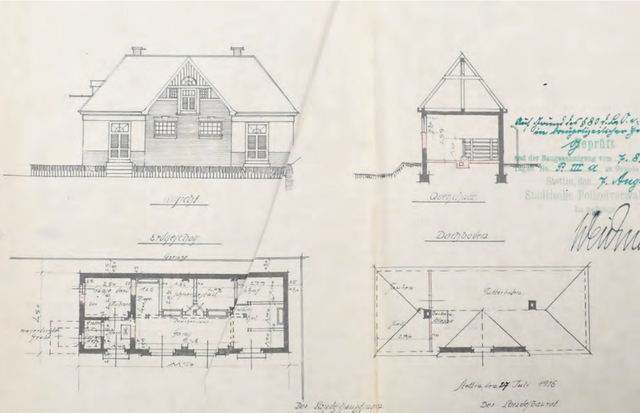
Rycina 26. Przebudowa obiektu pomocniczego przy Prowincjonalnym Zakładzie dla Głuchoniemych na cele hodowlane, 1916, APS, AMSPB, 204
