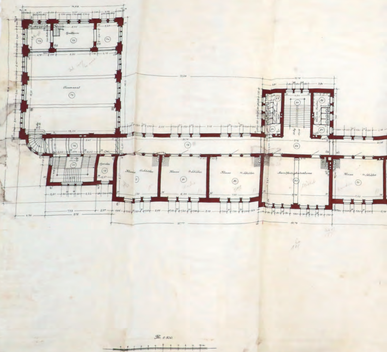
Rycina 24. Rzut parteru budynku, 1914, APS, AMSPB, 204
