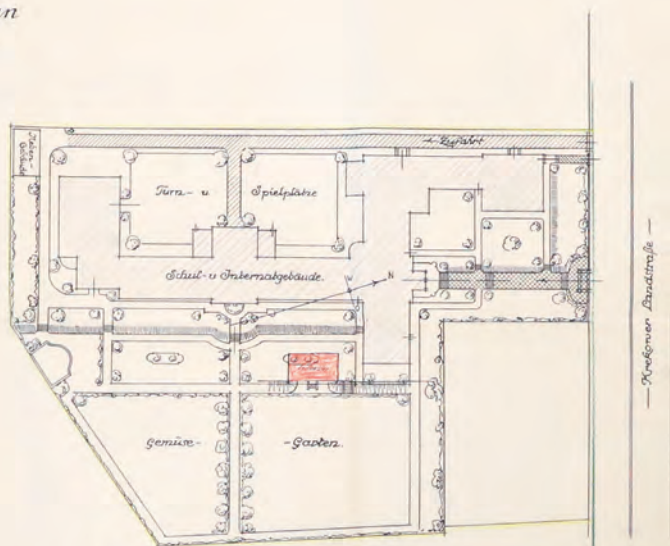
Rycina 27. Położenie budynku Prowincjonalnego Zakładu dla Głuchoniemych na parceli (na czerwono zaznaczona piwnica warzywna), 1919, APS, AMSPB, 204
