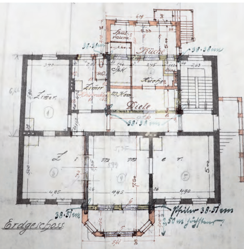
Rycina 74. Rzut parteru willi z dobudowaną werandą i przebudowaną kuchnią, 1917, APS, AMSPB, 4078
