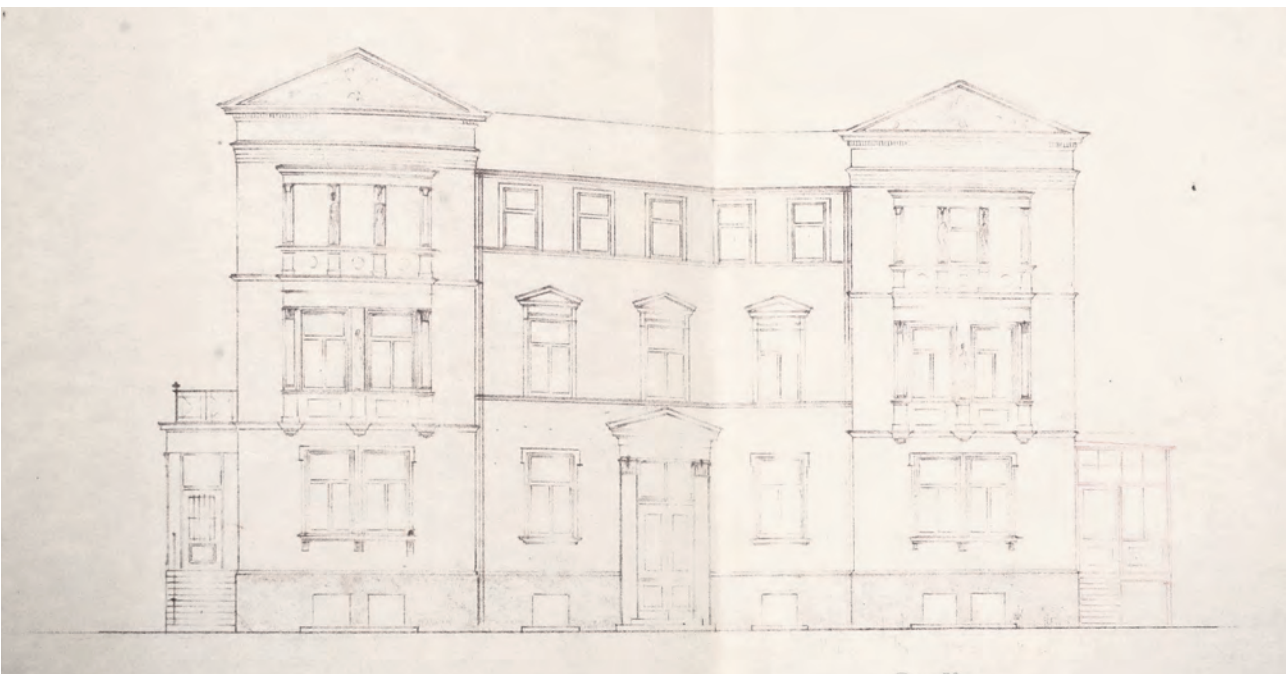
Rycina 56. Elewacja willi od strony ul. ks. Piotra Wawrzyniaka, 1932, APS, AMSPB, 6395
