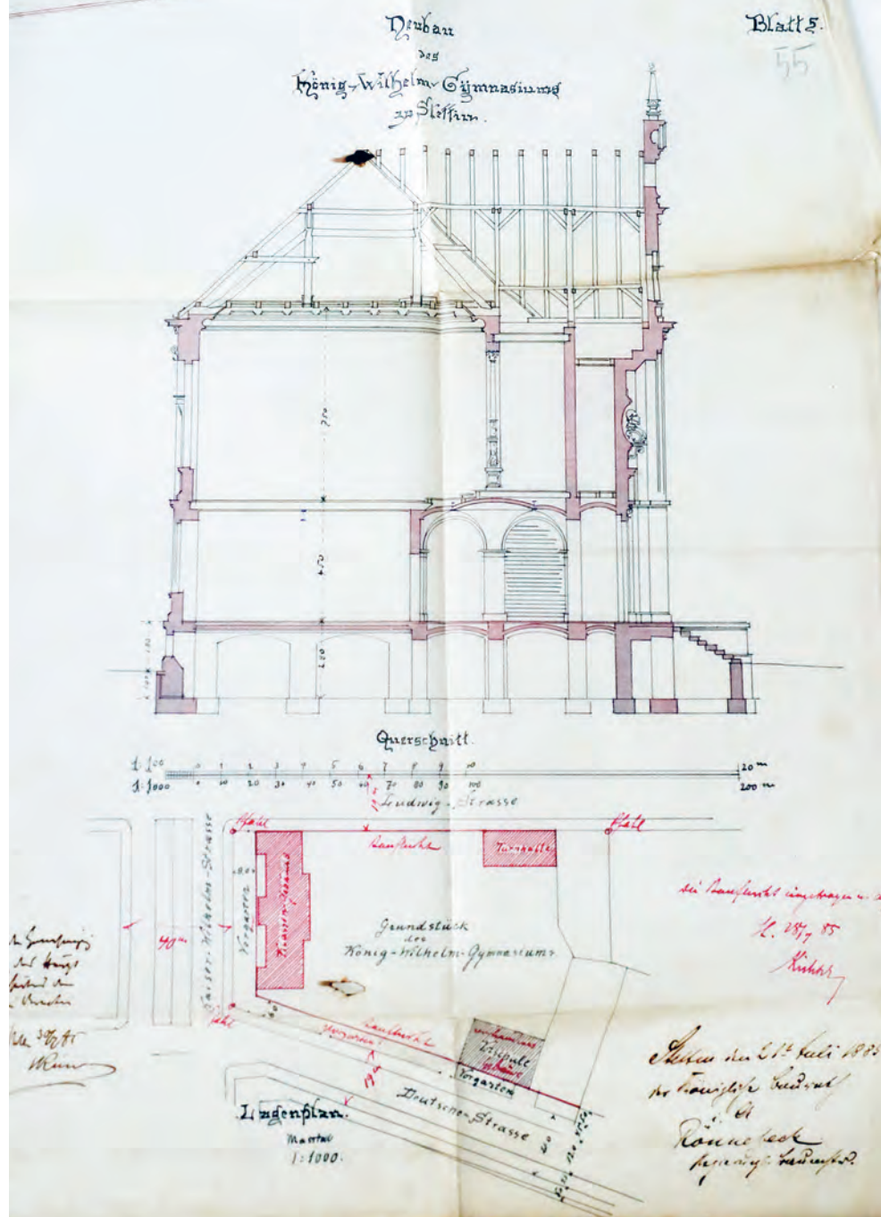
Rycina 6. Przekrój głównego budynku Gimnazjum Króla Wilhelma i położenie nowych obiektów na parceli, 1885 APS, AMSPB, 1185
