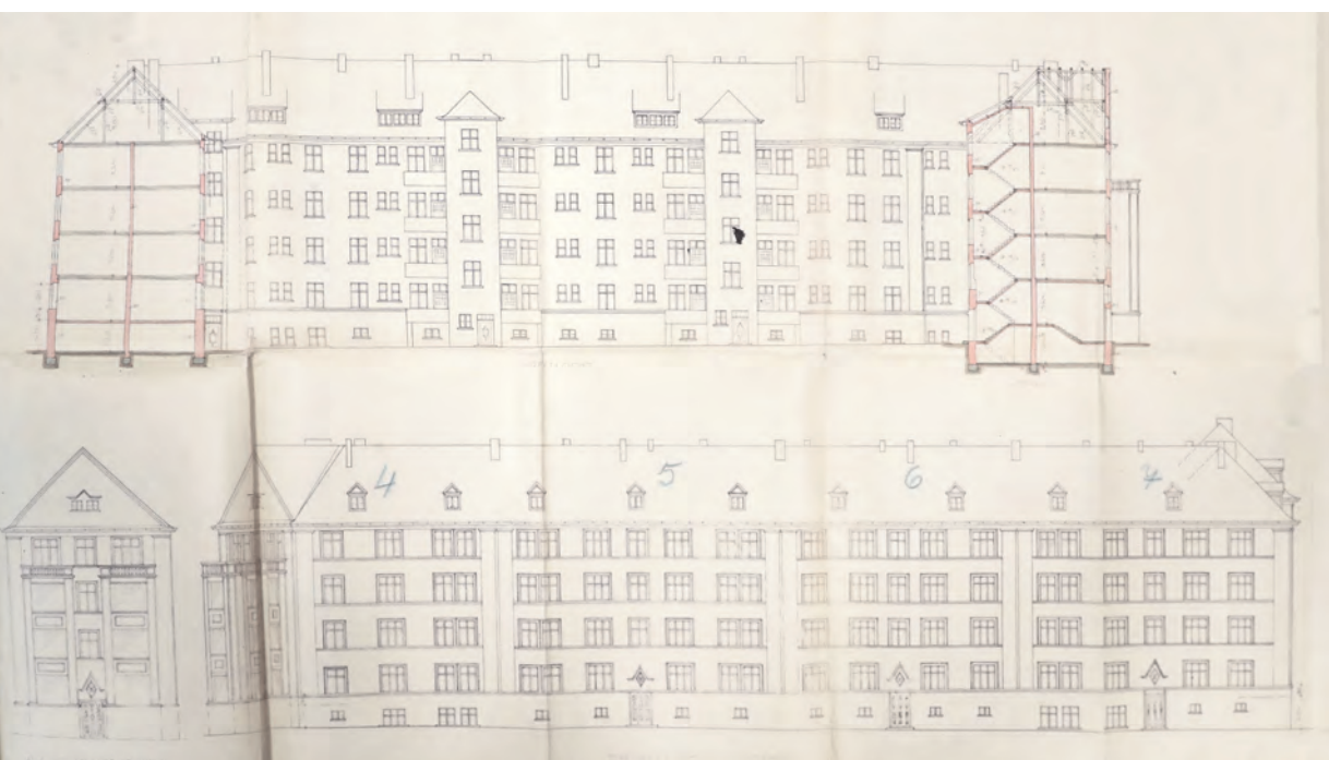
Rycina 65. Elewacja budynków mieszkalnych od strony podwórza i od al. Bohaterów Warszawy, 1928, APS, AMSPB, 9669
