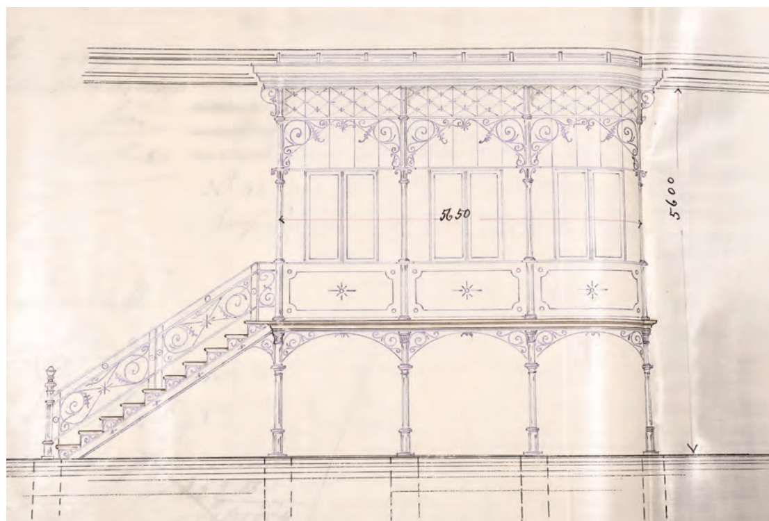
Rycina 53. Wejście boczne do willi dobudowane od strony północnej, 1888, APS, AMSPB, 6395
