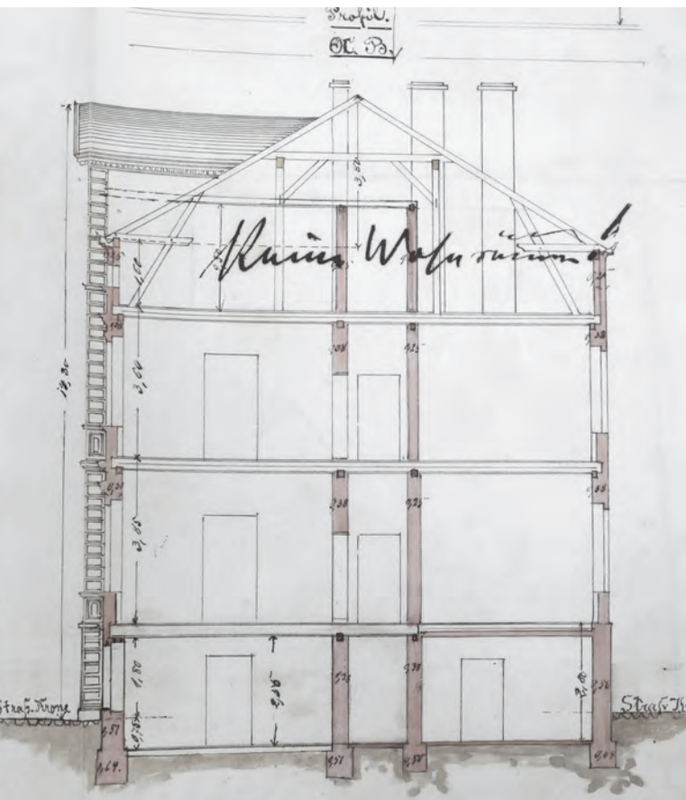
Rycina 68. Przekrój willi, 1881 APS, AMSPB, 4078
