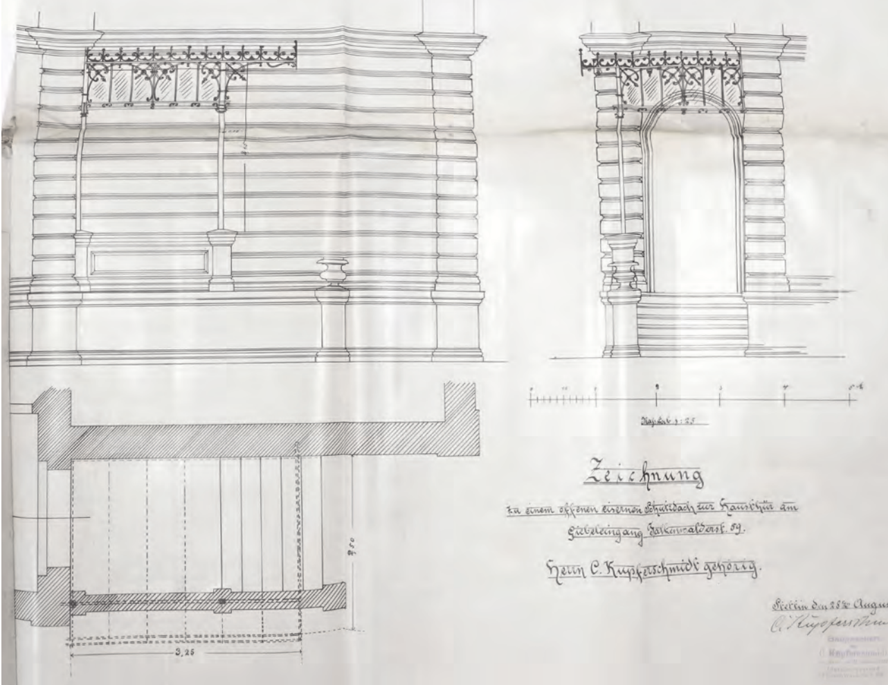
Rycina 77. Stalowy daszek nad wejściem do willei, 1900, APS, AMSPB, 4079
