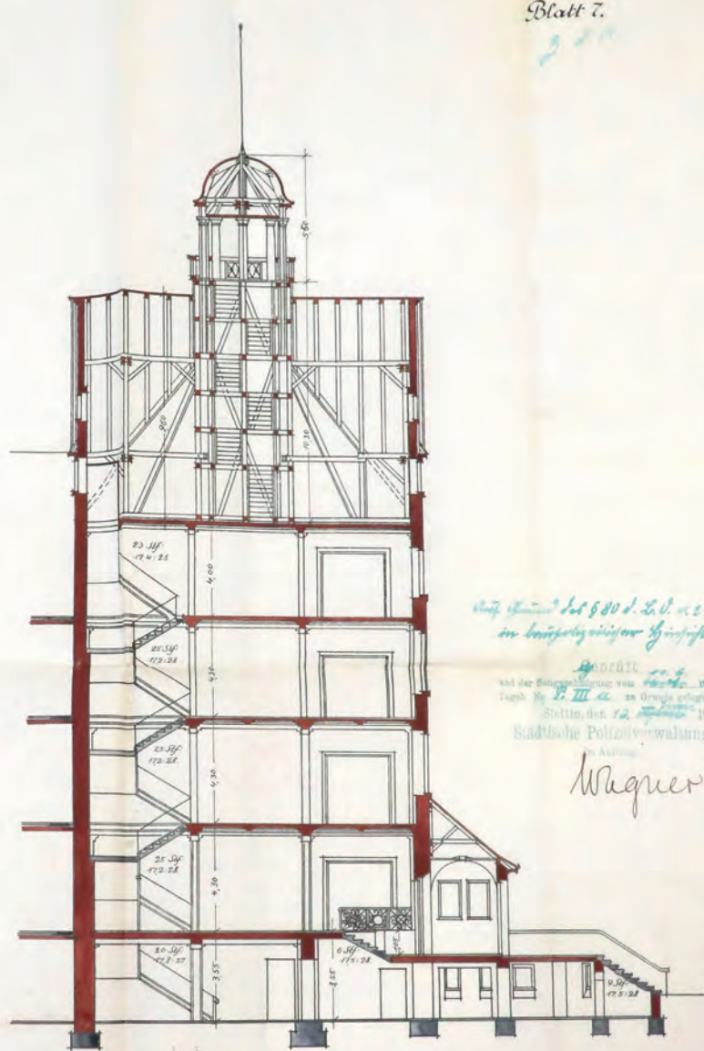
Schnitt: E - F.
