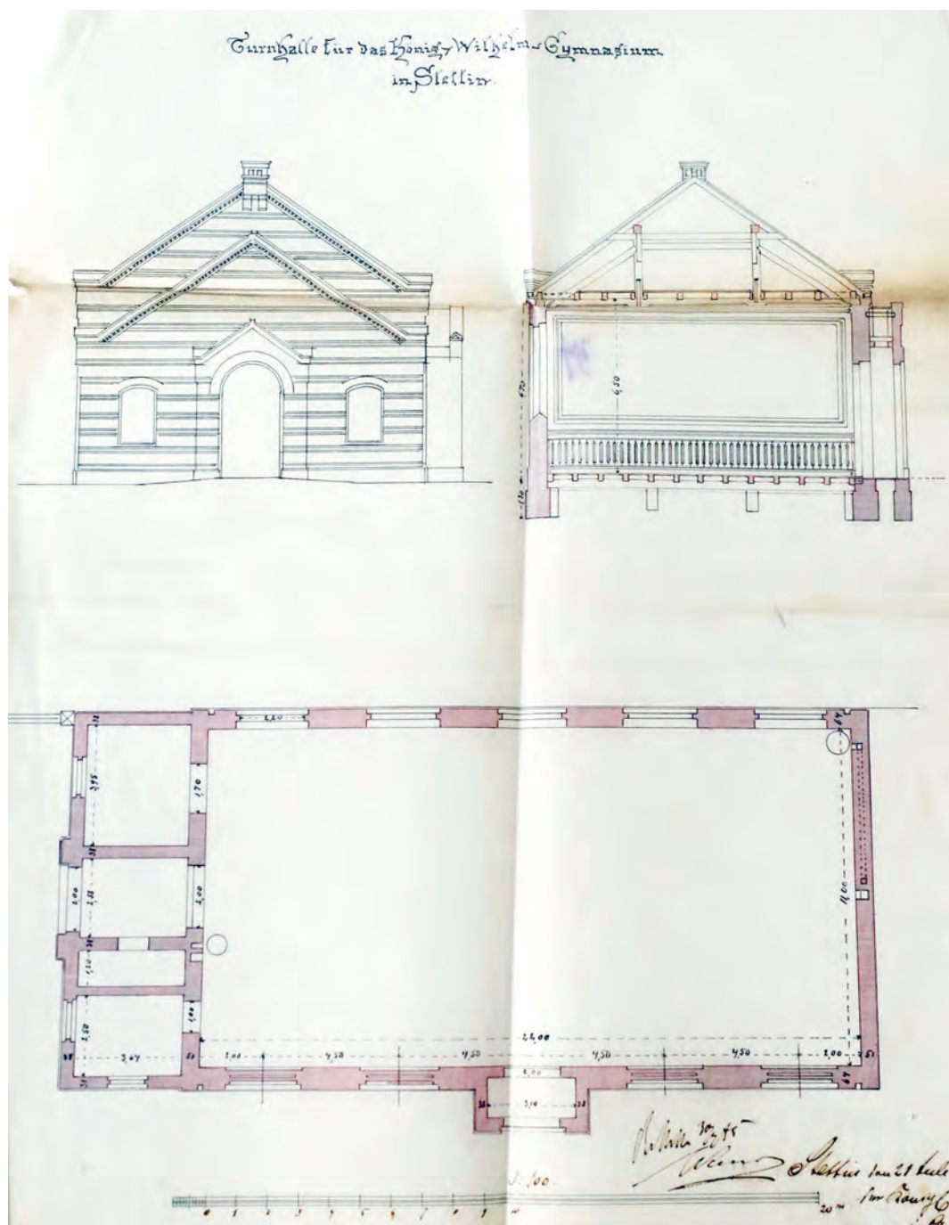
Rycina 8. Widok z boku, przekrój i rzut wolnostojącej sali gimnastycznej Gimnazjum Króla Wilhelma, 1885, APS, AMSPB, 1185
