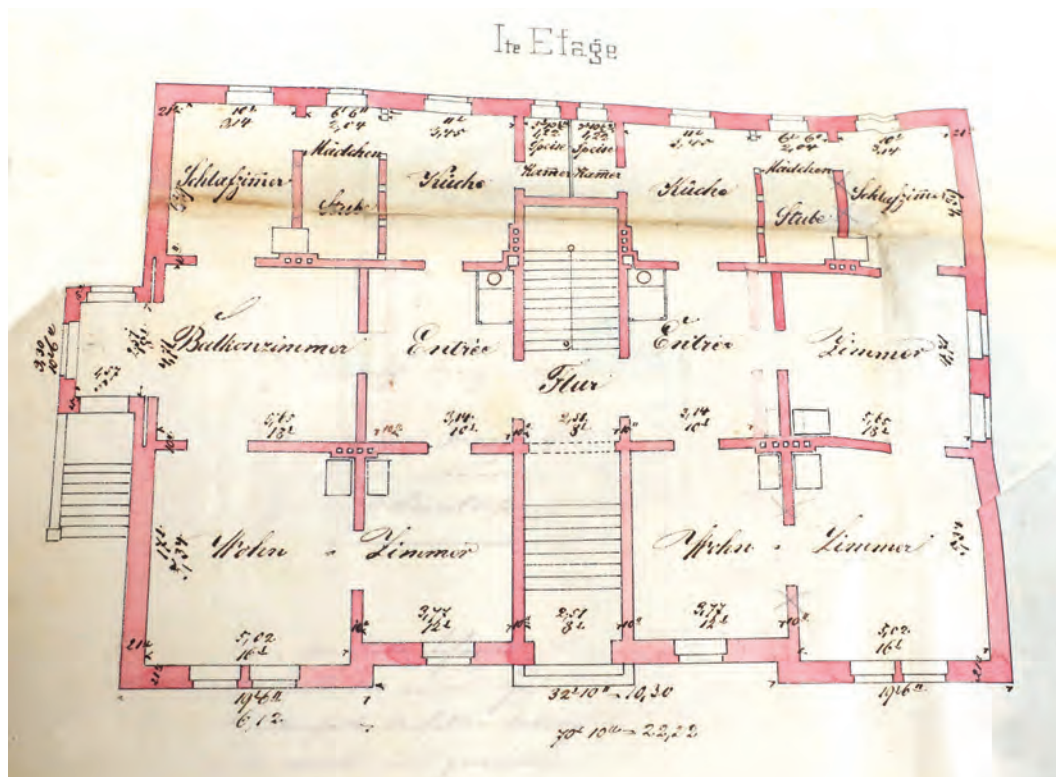
Rycina 51. Rzut pierwszego piętra willi z mieszkaniem, 1872, APS, AMSPB, 6395
