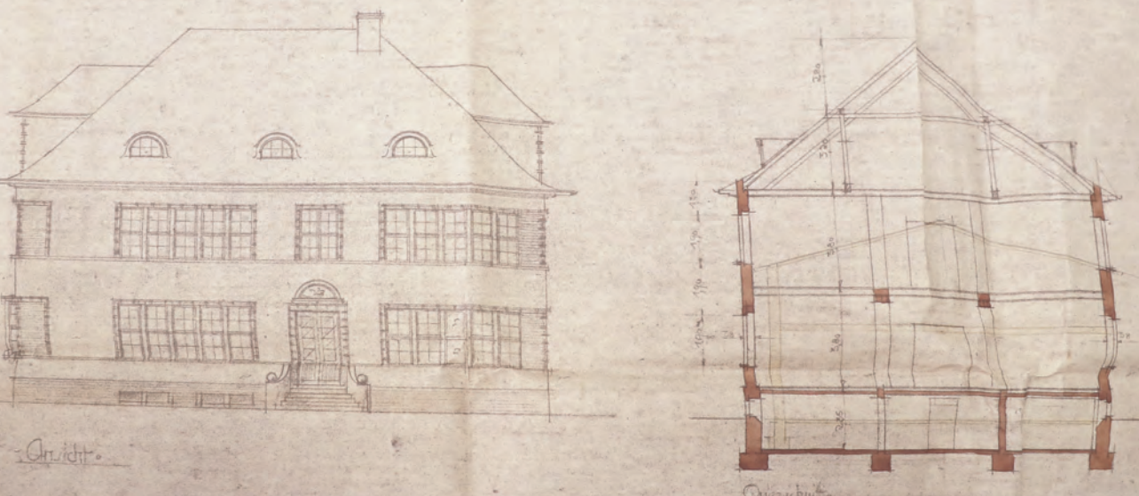
Rycina 92. Elewacja i przekrój nowego budynku na zapleczu szkoły dla dziewcząt Ernestinenhof, 1927 APS, AMSPB, 7900
