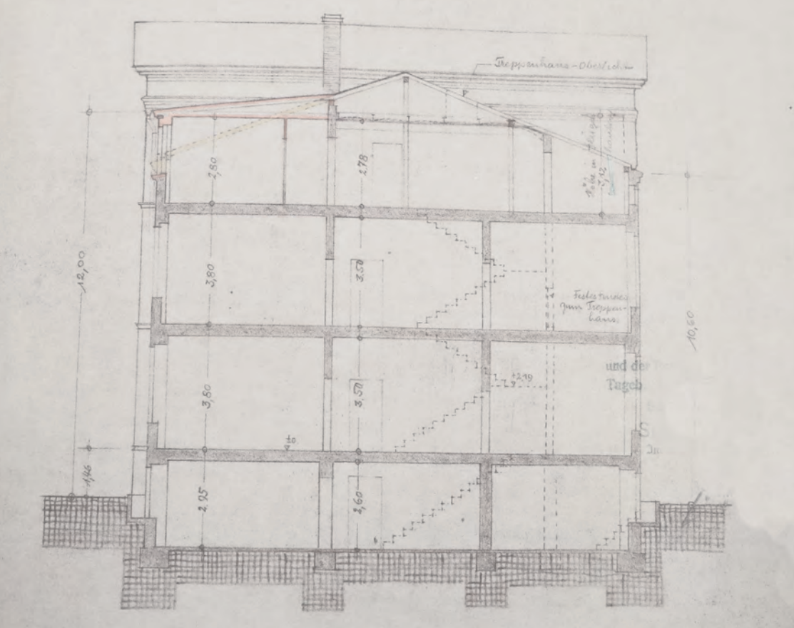
Rycina 58. Przekrój willi, 1932, APS, AMSPB, 6395
