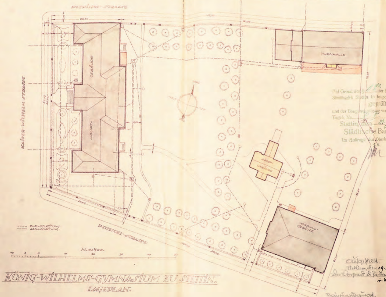
Rycina 9. Położenie na parceli wszystkich obiektów Gimnazjum Króla Wilhelma, 1936 APS, AMSPB, 1185
