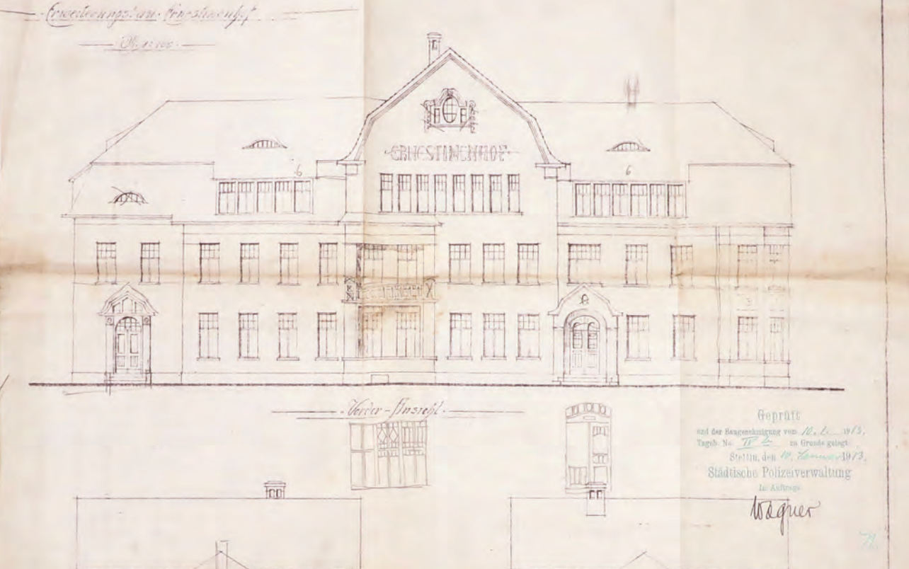
Rycina 88. Elewacja przebudowanej szkoły dla dziewcząt Ernestinenhof, 1913, APS, AMSPB, 7900
