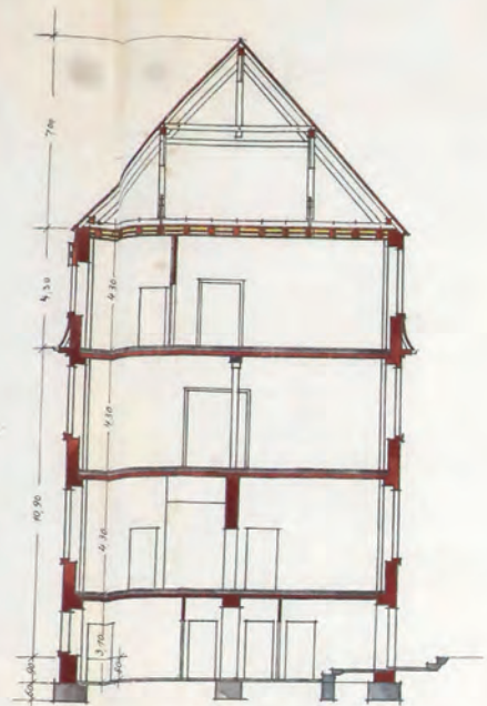
Schnitt: G - S.
