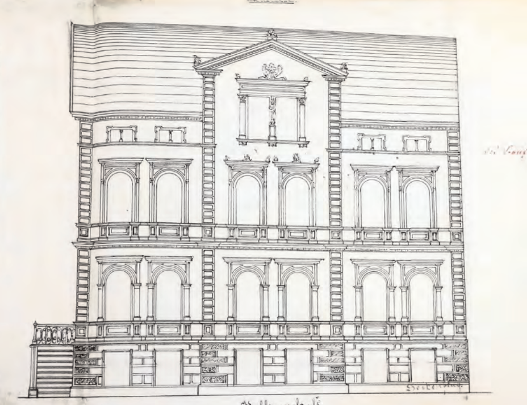
Rycina 67. Elewacja willi Kupferschmidta od strony al. Wojska Polskiego (nr 107), 1881 APS, AMSPB, 4078
