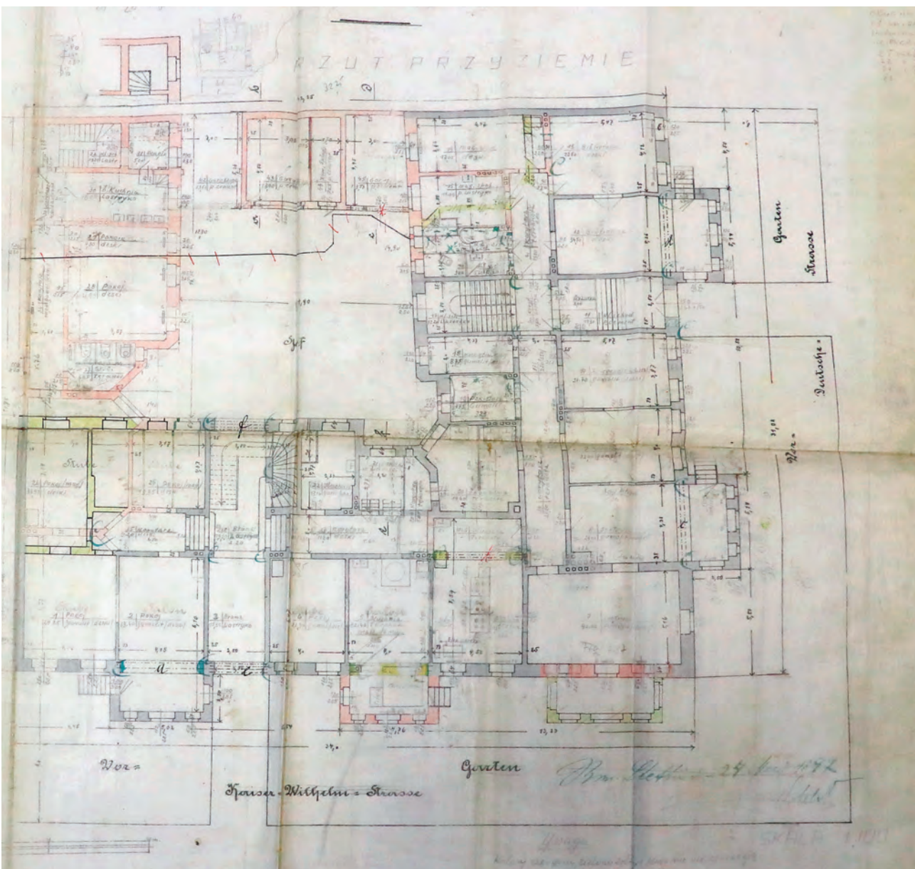
Rycina 18. Rzut parteru kamienicy po przeróbkach, 1897, APS, AMSPB, 48
