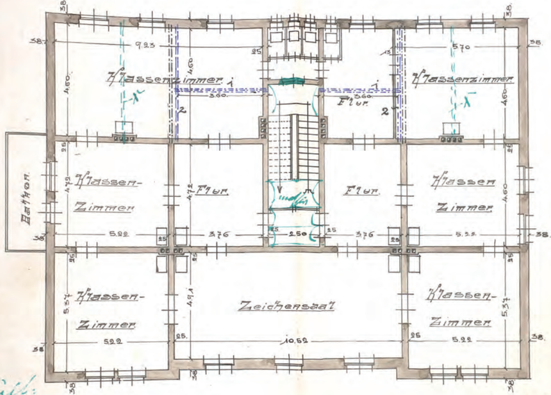
Rycina 54. Rzut pierwszego piętra willi z zatwierdzoną przebudową na potrzeby szkolne, 1906 APS, AMSPB, 6395
