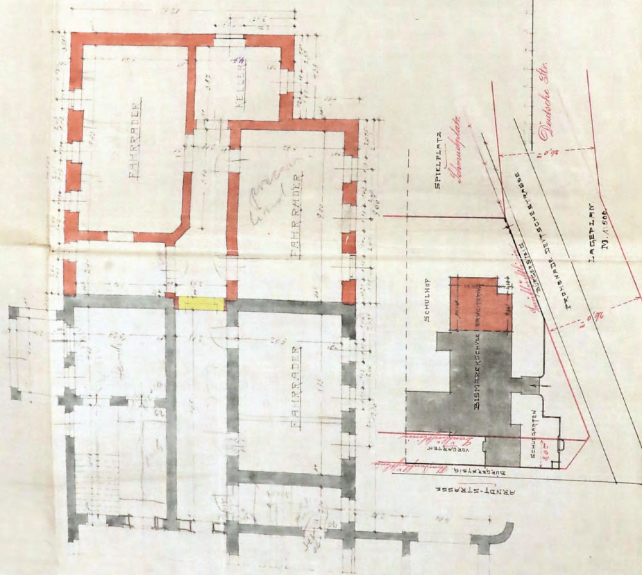
Rycina 41. Rzut piwnic i parteru dobudowanej części Gimnazjum Realnego im. Ottona Bismarcka, 1912, APS, AMSPB, 4601
