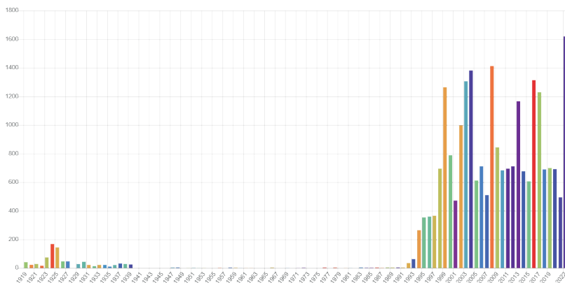
Wykres 2. Frekwencja połączenia język polski w KDP w latach 1918–2023
