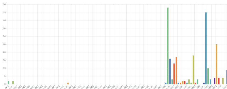
Wykres 11. Frekwencja połączenia język słowacki w KDP w latach 1918–2023
