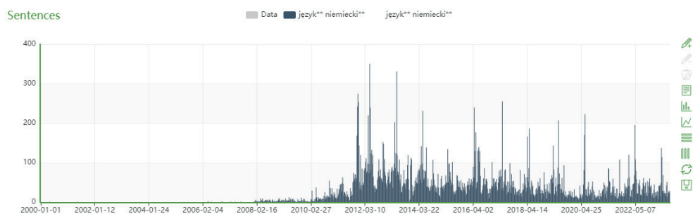
Wykres 7. Frekwencja połączenia język niemiecki w Monco Pl w latach 2010–2023
