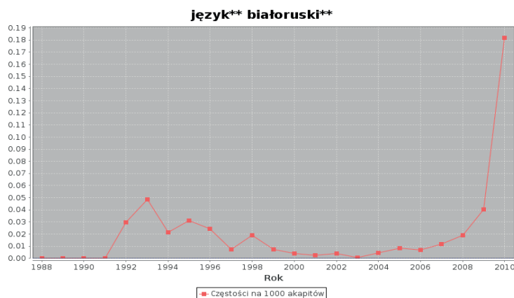
Wykres 18. Frekwencja połączenia język białoruski w NKJP w latach 1988–2010
