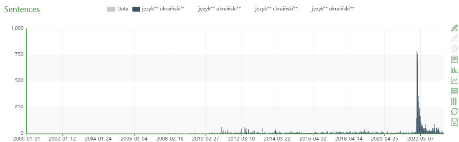
Wykres 16. Frekwencja połączenia język ukraiński w Monco.pl w latach 2010–2023 Źródło: Monco.pl.
