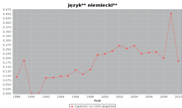
Wykres 6. Frekwencja połączenia język niemiecki w NKJP w latach 1988–2010
