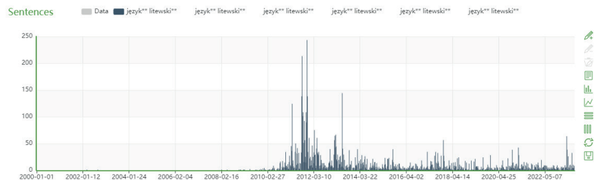
Wykres 22. Frekwencja połączenia język litewski w Monco.pl w latach 2010–2023
