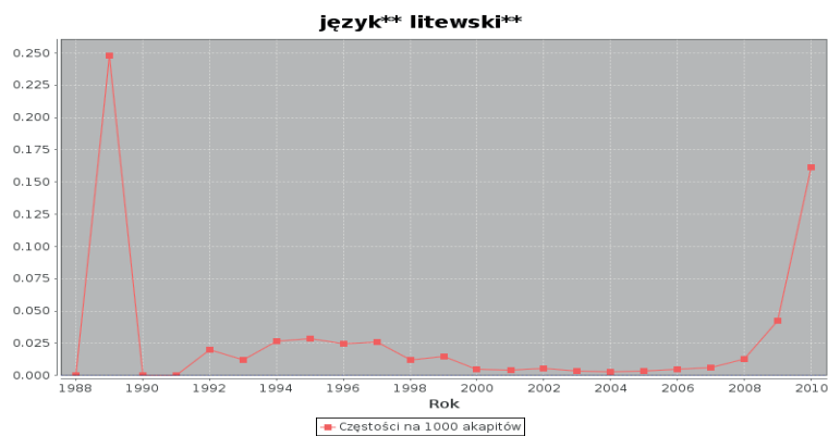
Wykres 21. Frekwencja połączenia język litewski w NKJP w latach 1988–2010
