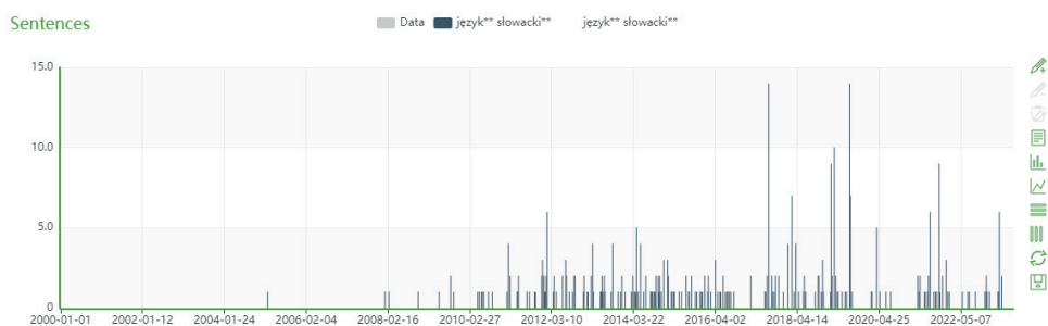
Wykres 13. Frekwencja połączenia język słowacki w Monco Pl w latach 2010–2023
