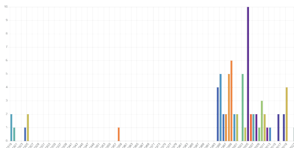
Wykres 8. Frekwencja połączenia język czeski w KDP w latach 1918–2023
